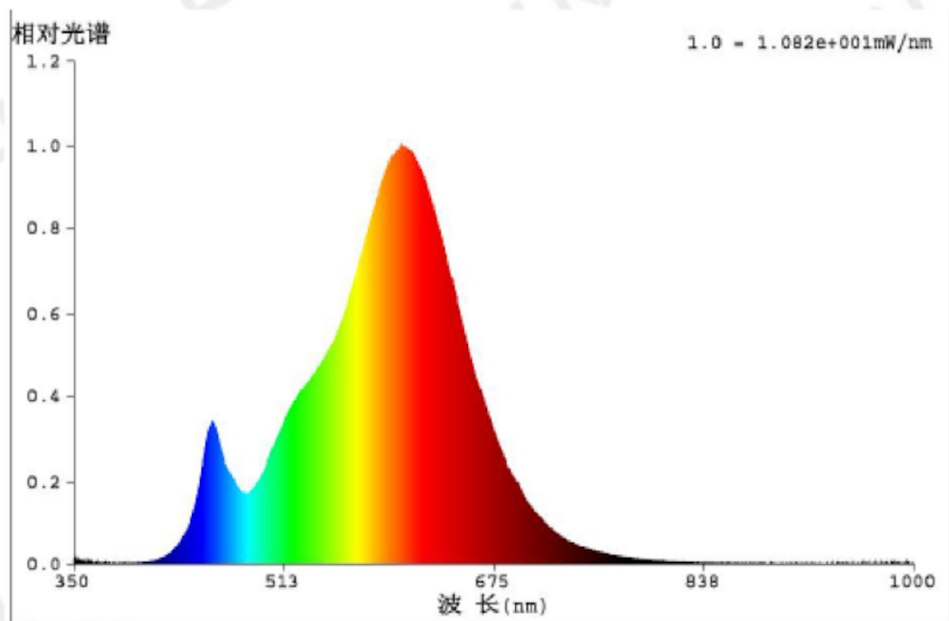
光谱分布
